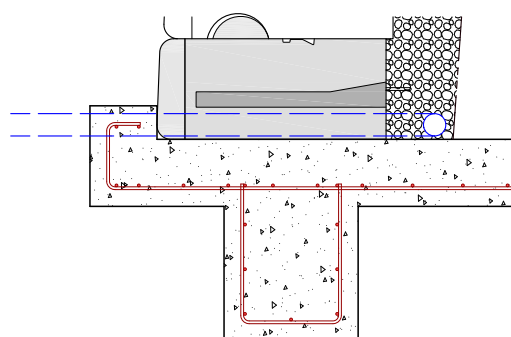
D. Semelle de fondation en béton armé
